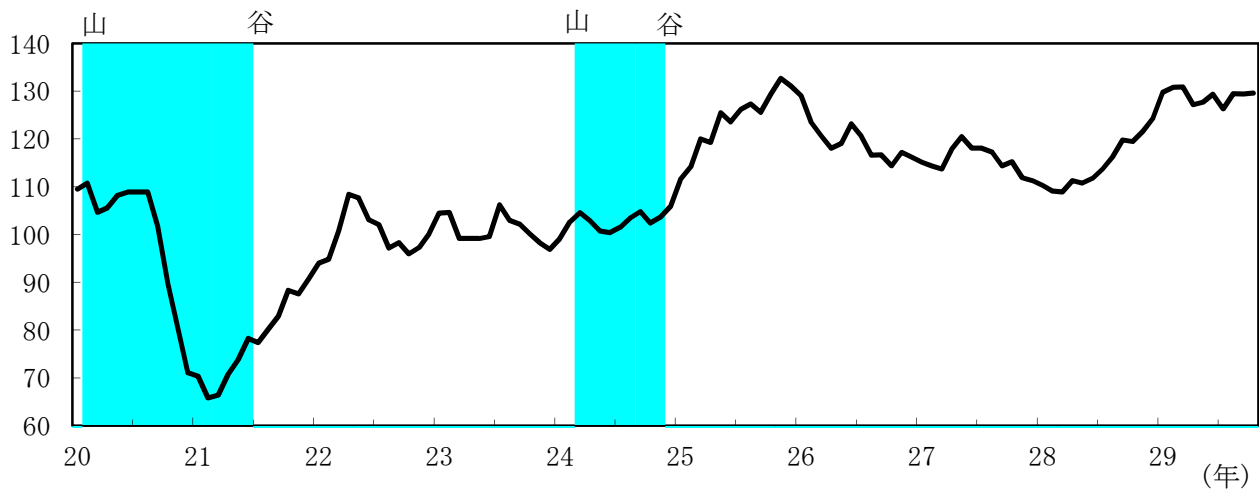
(2) 一致指数
